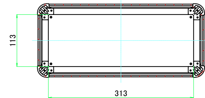
C-C ( 1 : 5 )
