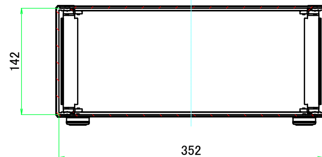
A-A ( 1 : 5 )
